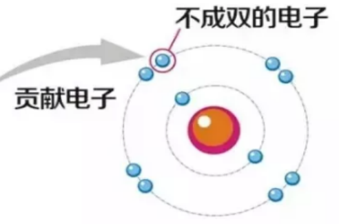
自由基
